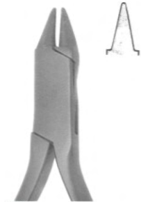
2703 ADAMS (Fig. 44) 12.5 cm, 5" Sling clasp & wire bending plier.
