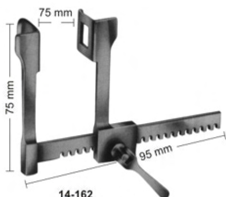
14-162 FINOCHIETTO Blades 18X21 mm
