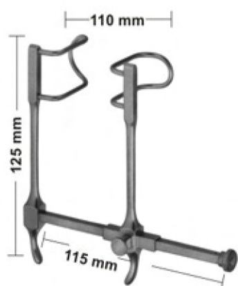
06-255 GOSSET Blades:38 mm deep
